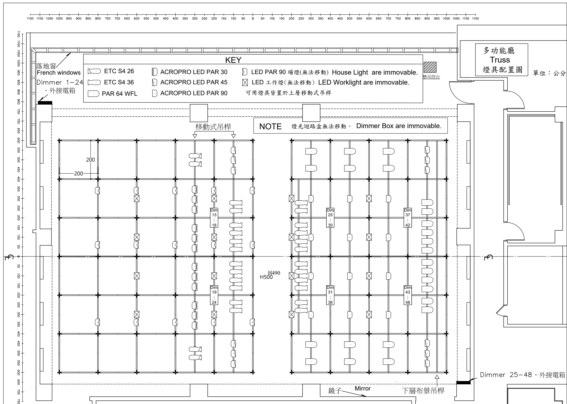
圖 (二) 多功能廳 桁架結構尺寸圖與燈具配置圖 (單位：公分) Figure(2) Multi Hall Grid Structure Size and Light Plot (upper layer) (Unit: cm)
