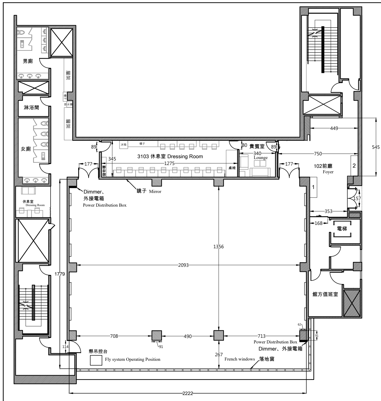
圖 (一) 多功能廳_平面圖 (單位: 公分) Figure(1) Multi Hall_Floor Plan (Unit: cm)
